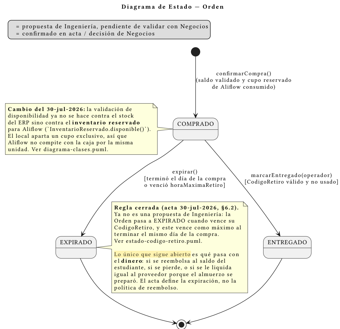
Figure 10: Estado: Orden
