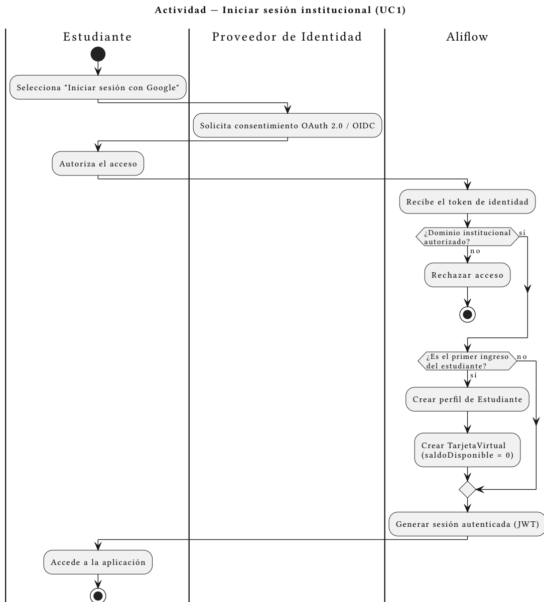
Figure 1: Actividad: autenticación
