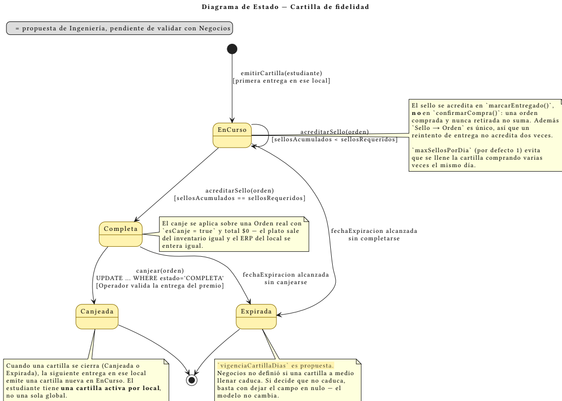
Figure 14: Estado: Cartilla
