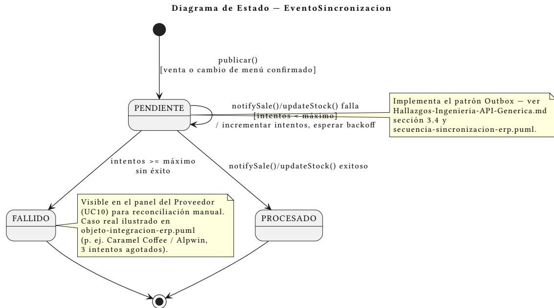
Figure 13: Estado: EventoSincronizacion
